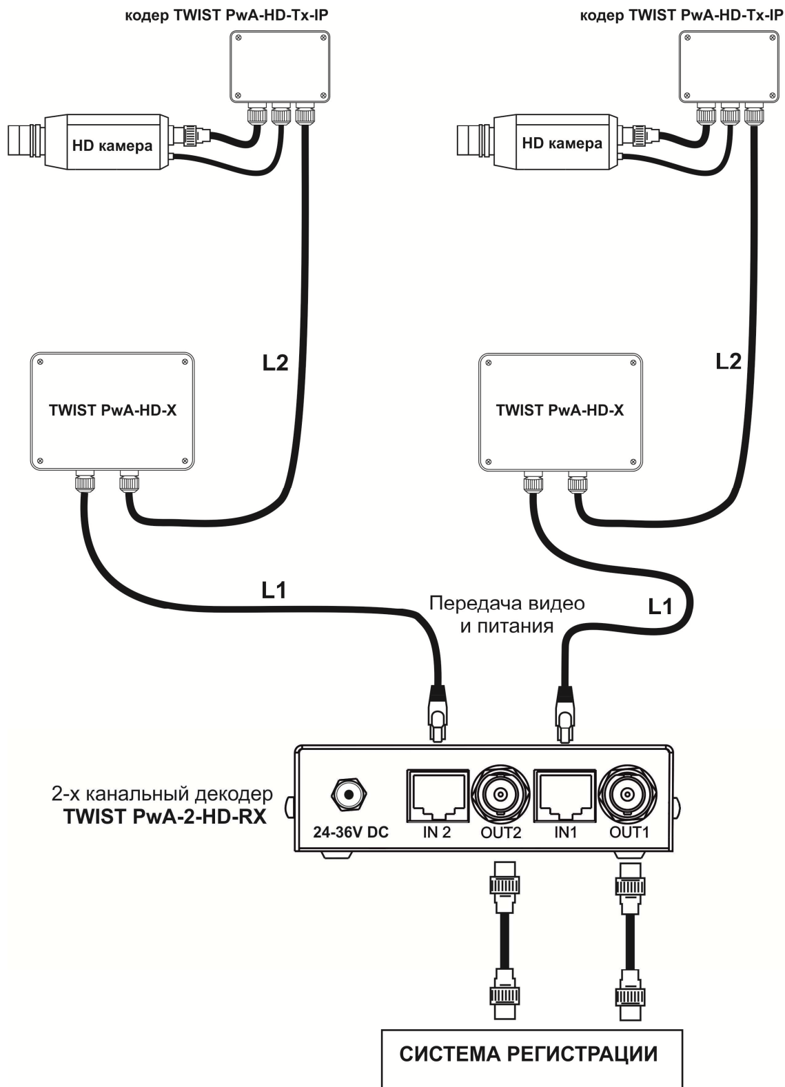
Рис.2 Схема подключения TWIST PwA-HD-X для ретрансляции видеосигнала.
