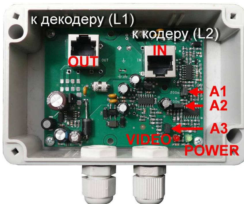
Рис.1 Внешний вид и схема внутреннего подключения TWIST PwA-HD-X.
