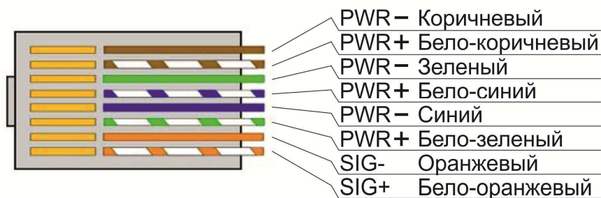
Рис.3 Обжим витой пары.
